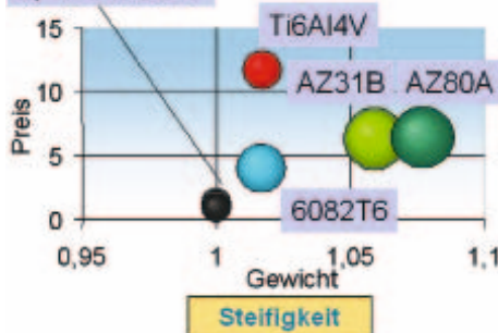
Zugstäbe unter gleicher Last, entweder auf gleiche elastische Dehnung oder Festigkeit dimensioniert. Bild: Hirschvogel
